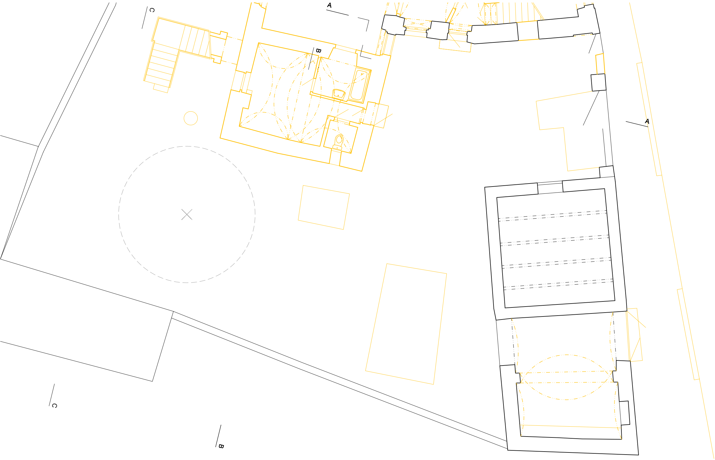
PŮDORYS 1.NP / SOUČASNÝ STAV A BOURANÉ KONSTRUKCE
